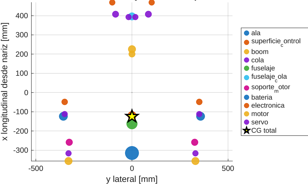
Distribucion de masa y CG - vista superior
